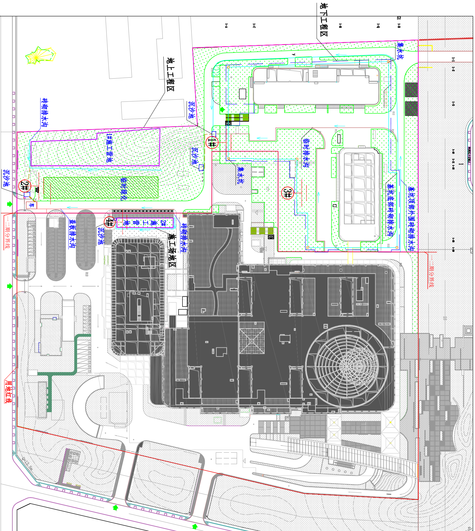
附图2 防治责任范围、监测分区及监测点布设图
